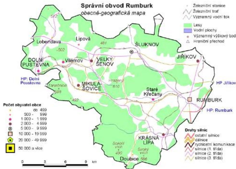
Obrázek 2: Dopravní infrastruktura v Šluknovském výběžku
