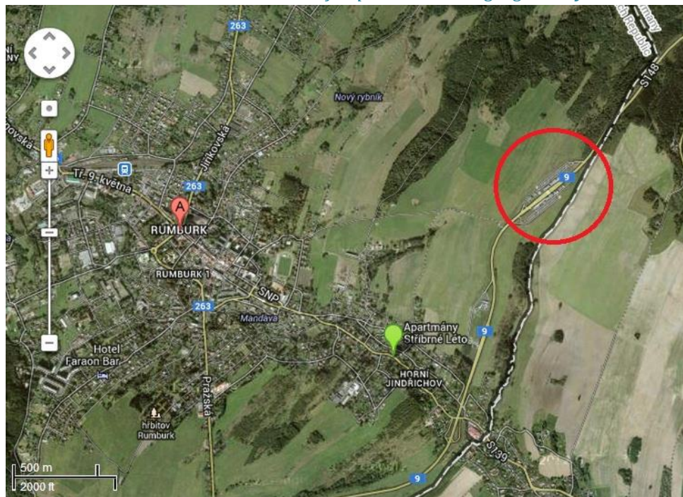
Obrázek 6: Satelitní snímek znázorňující prostorovou segregaci ubytoven „Na svahu“ a „V2“
