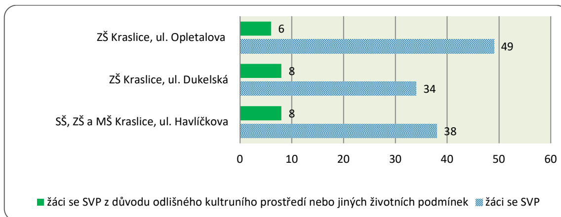
Graf 6. Žáci se SVP a žáci se SVP z důvodu odlišného kulturního prostředí a jiných životních podmínek v kraslických základních školách k 30. 9. 2018
